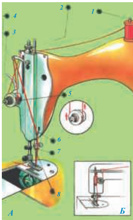
Расми 43. Пайдарҳамии гузаронидани риштаи болоӣ дар мошини дарздӯзии дастӣ
