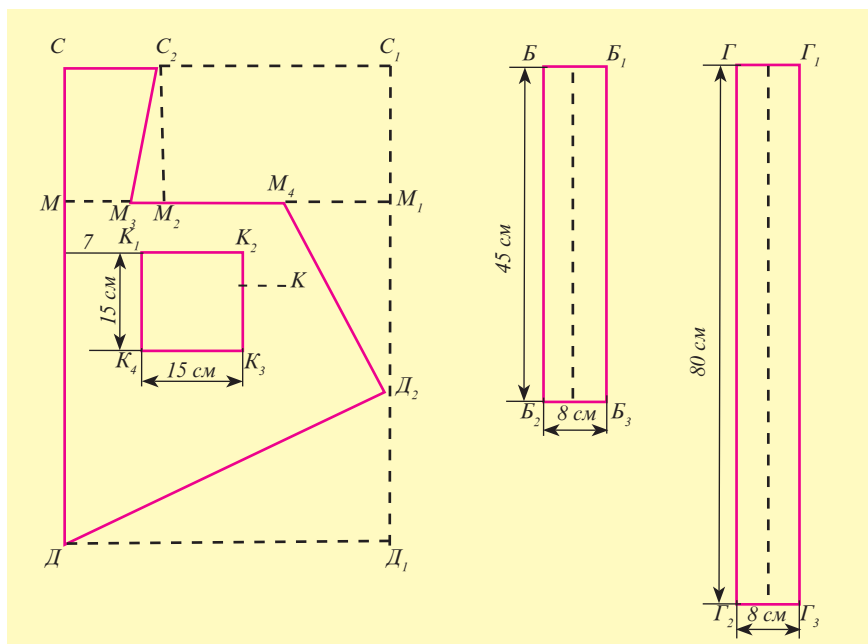
Расми 68. Нақшаи пешдомани оройишӣ
